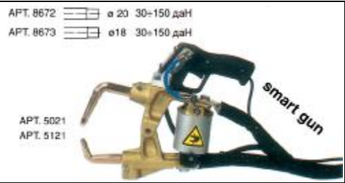
Smart gun: Клещи пневматические с воздушным (Арт. 8672) и водяным (Арт. 8673) охлаждением. Возможность использования: стандартные плечи и плечи с большим раствором. Арт. 5001...5085 и Арт. 5121...5185.
