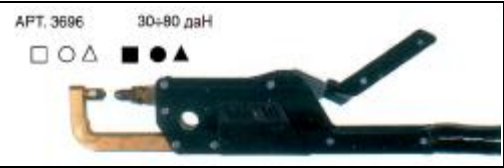
Клещи ручные типа «С» с воздушным охлаждением, малогабаритные. Длина кабелей 1600 мм.
