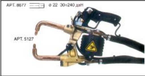
Smart gun: Клещи пневматические с водяным охлаждением. Возможность использования: стандартные плечи и плечи с большим раствором Арт. 5127...5137.
